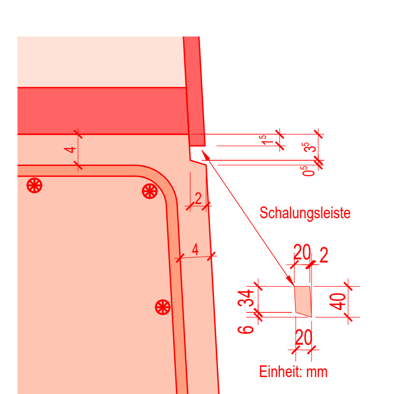
Detail -A-, 1 : 5
