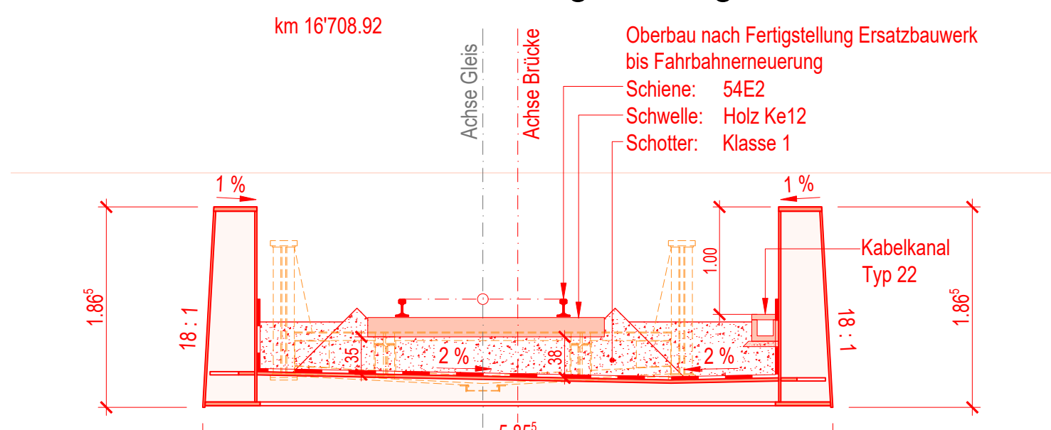
Querschnitt -3- nach Fertigstellung, 1 : 50
