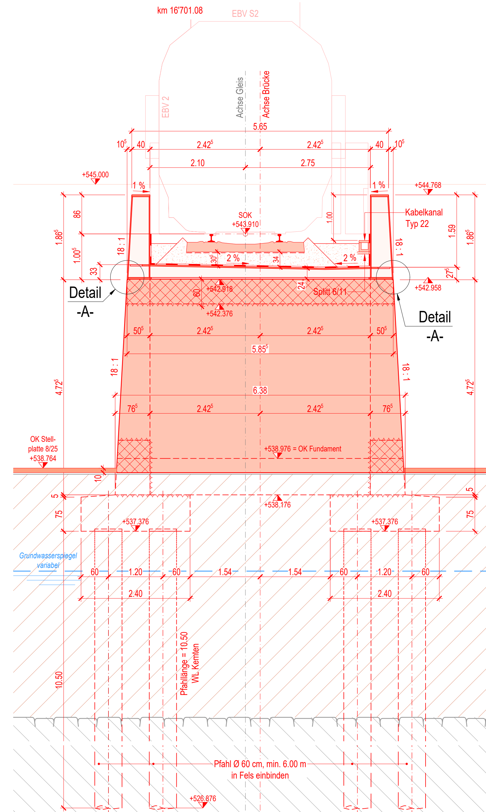
Querschnitt -4-, 1 : 50
