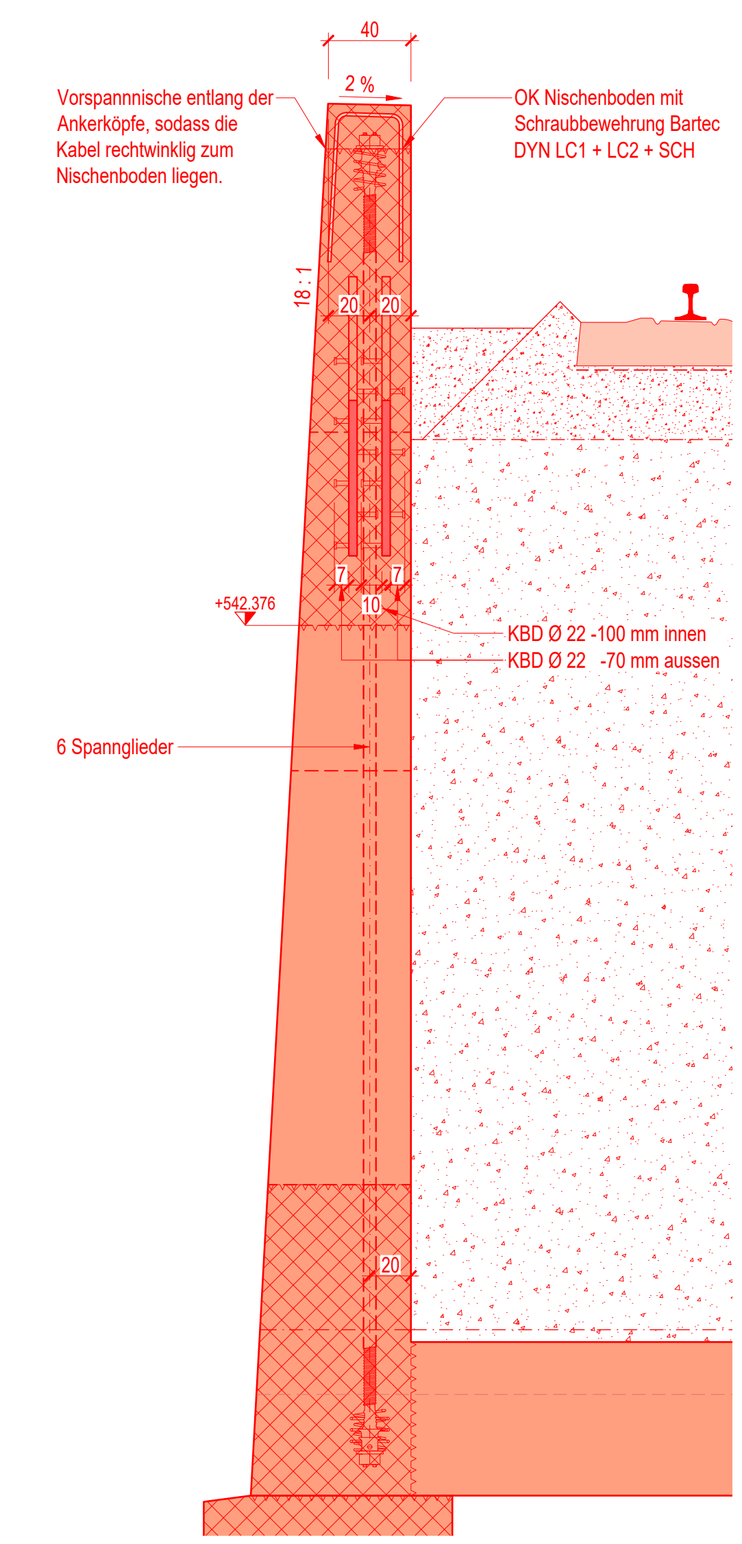
Detail -C- Querschnitt, 1 : 25
