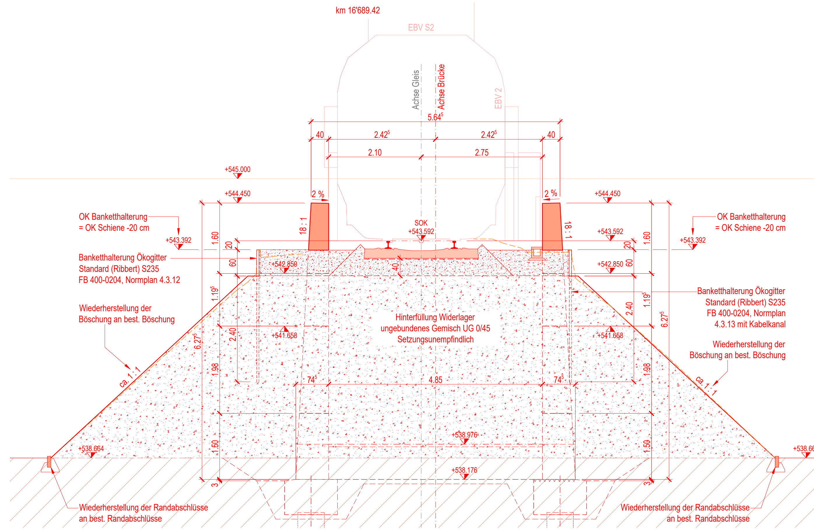
Querschnitt -8-, 1 : 50
