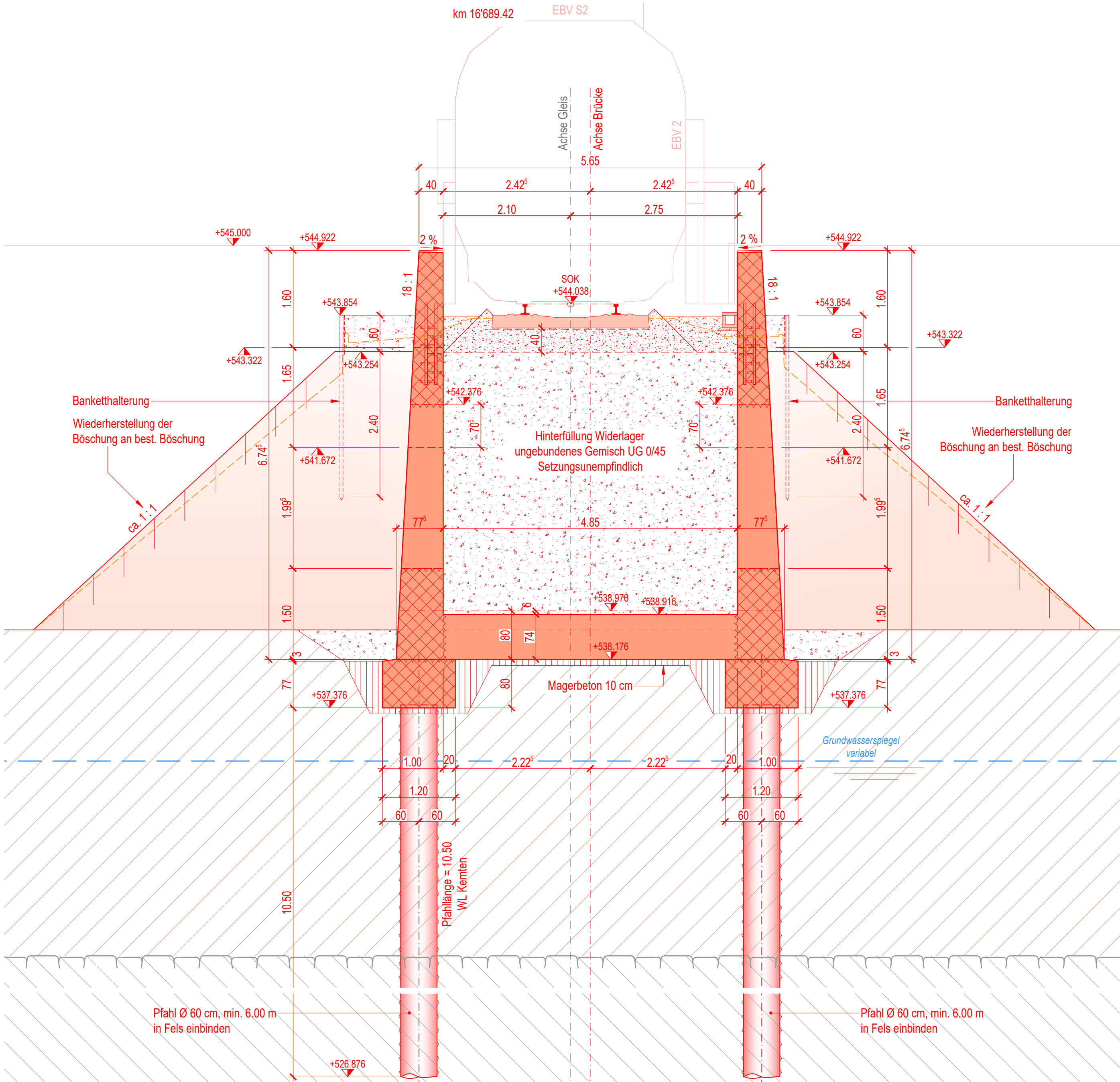
Querschnitt -6-, 1 : 50
