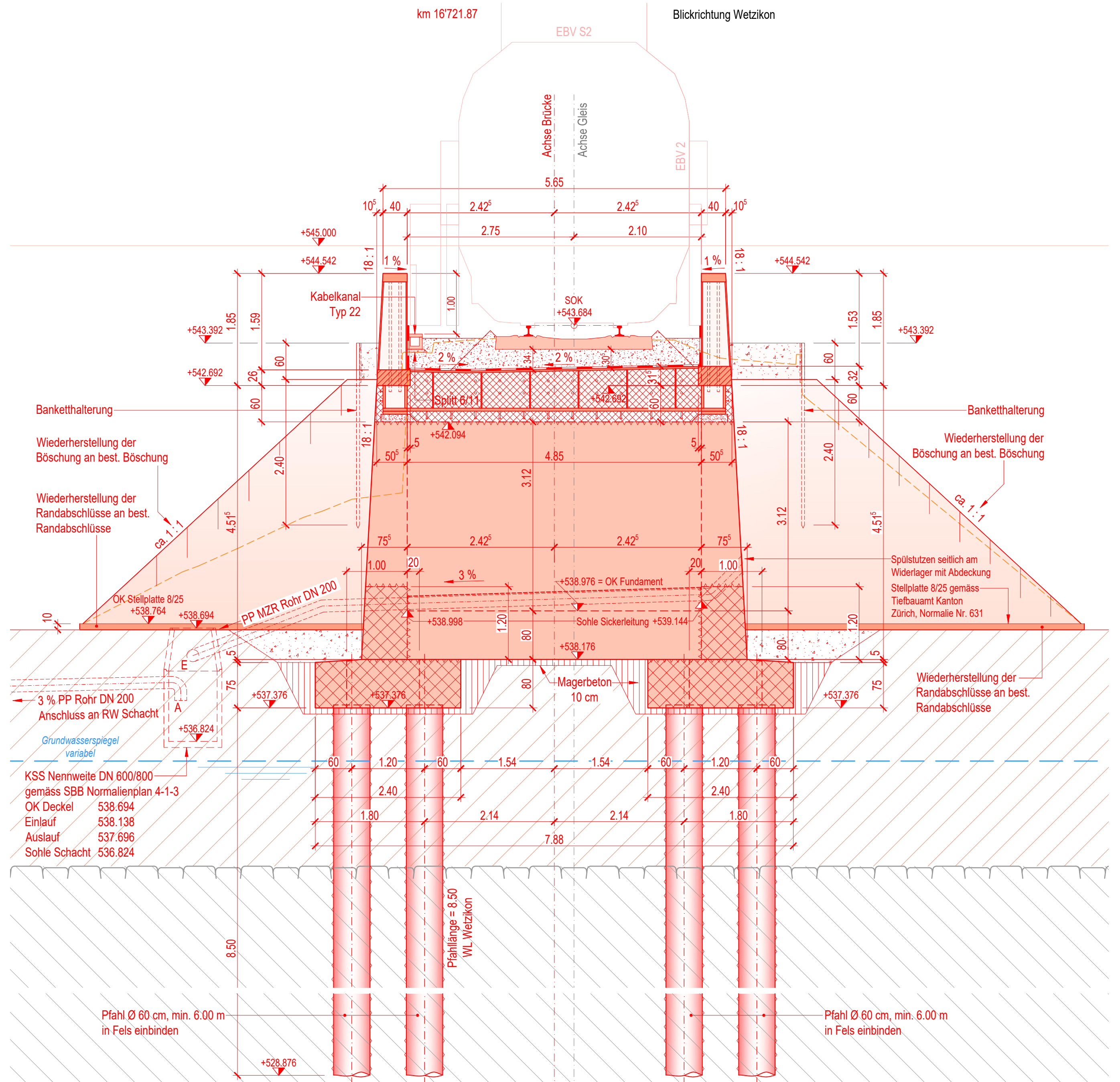
Querschnitt -7-, 1 : 50
