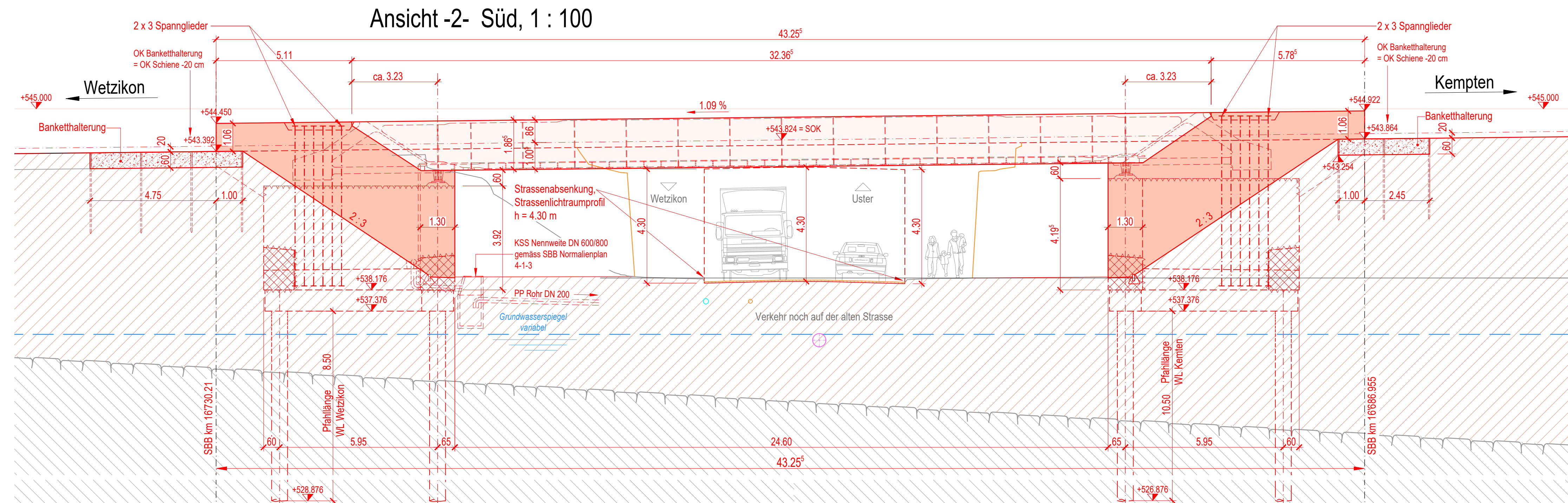
Ansicht -2- Süd, 1 : 100
