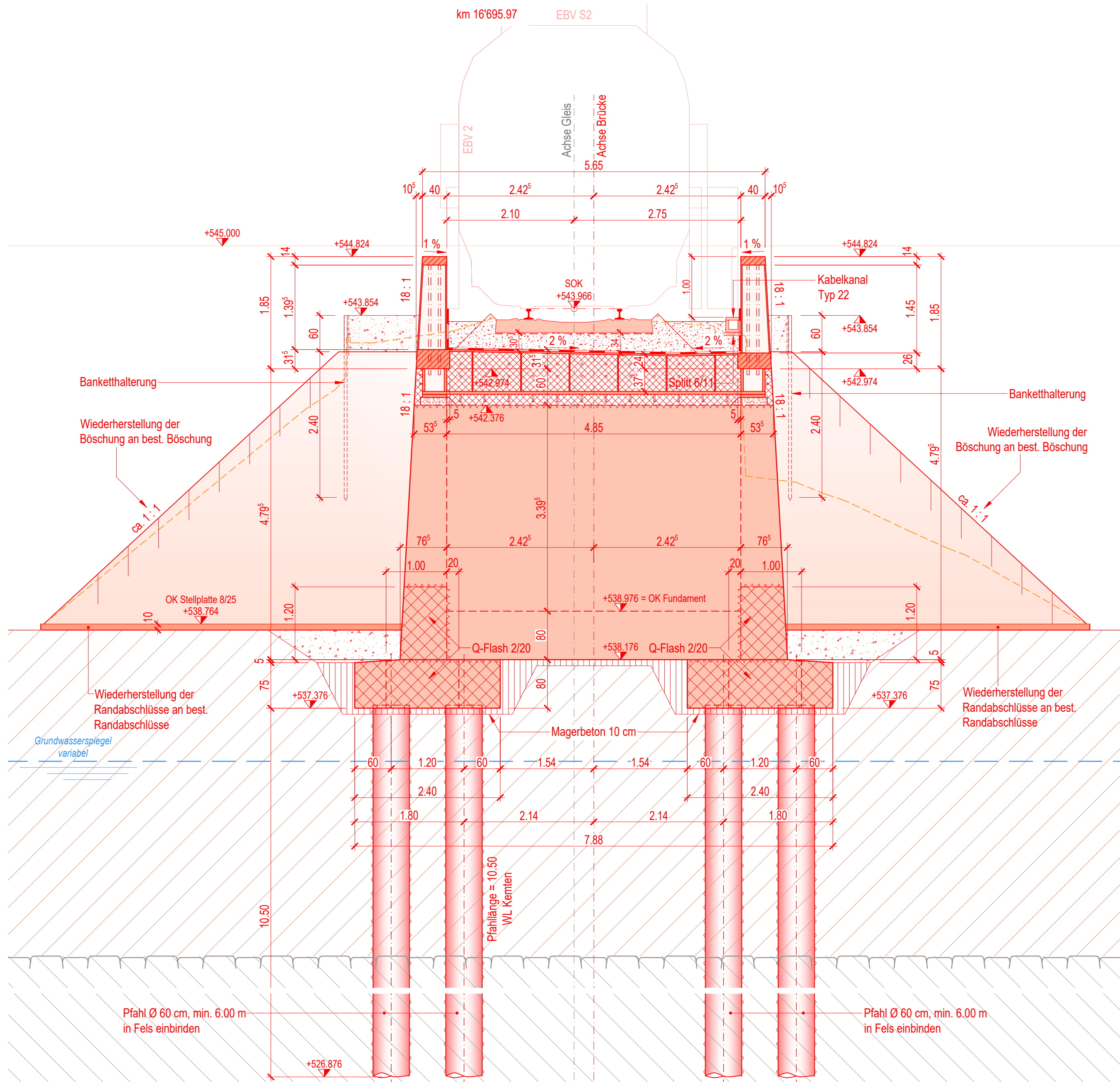
Querschnitt -5-, 1 : 50
