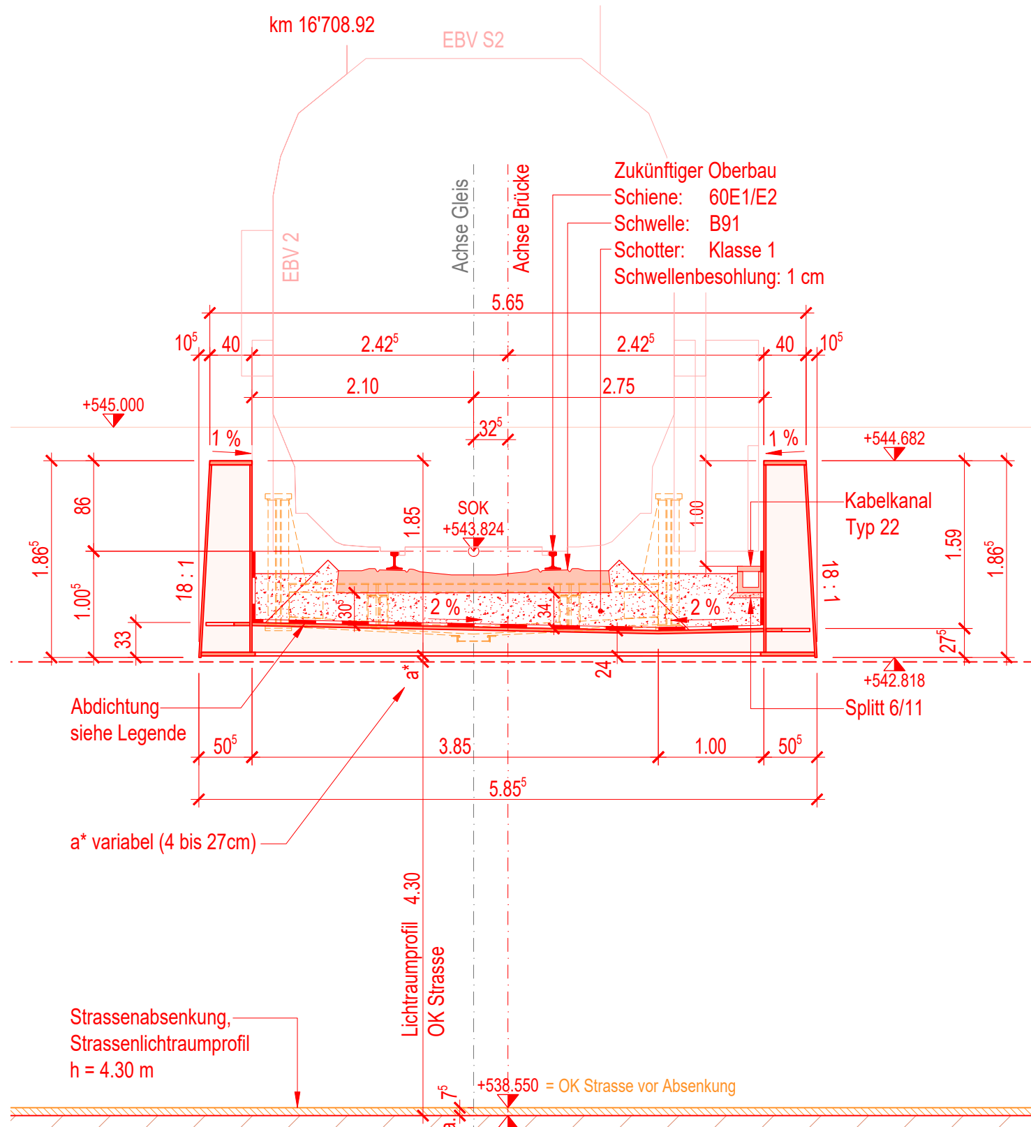
Querschnitt -3-, 1 : 50
